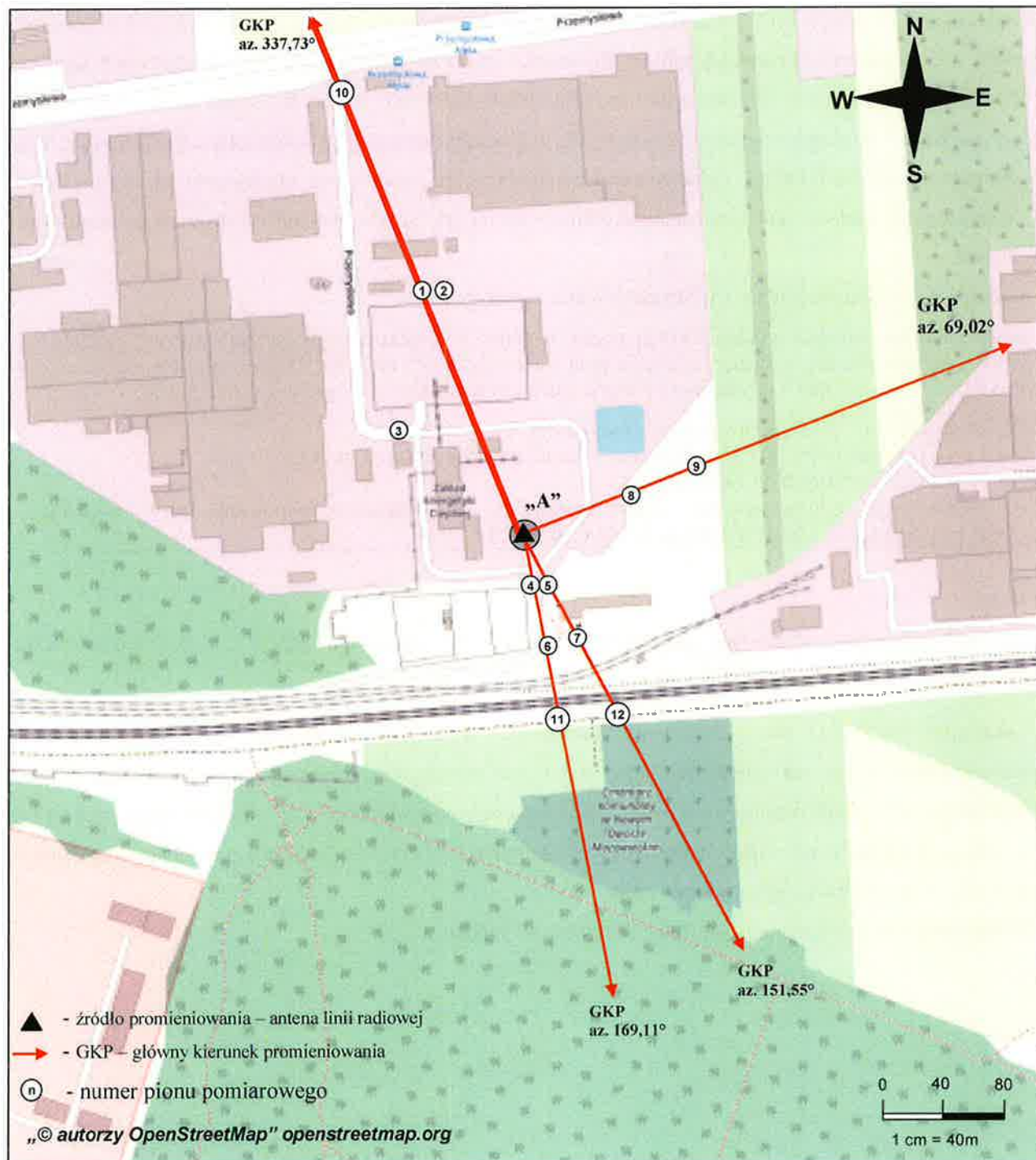
Rys. 1. Usytuowanie punktów i pionów pomiarowych w otoczeniu instalacji radiokomunikacyjnej Stacja Netia NDWMB001 - NDWMM00002 Nowy Dwór Mazowiecki, ul. Przemysłowa 1
